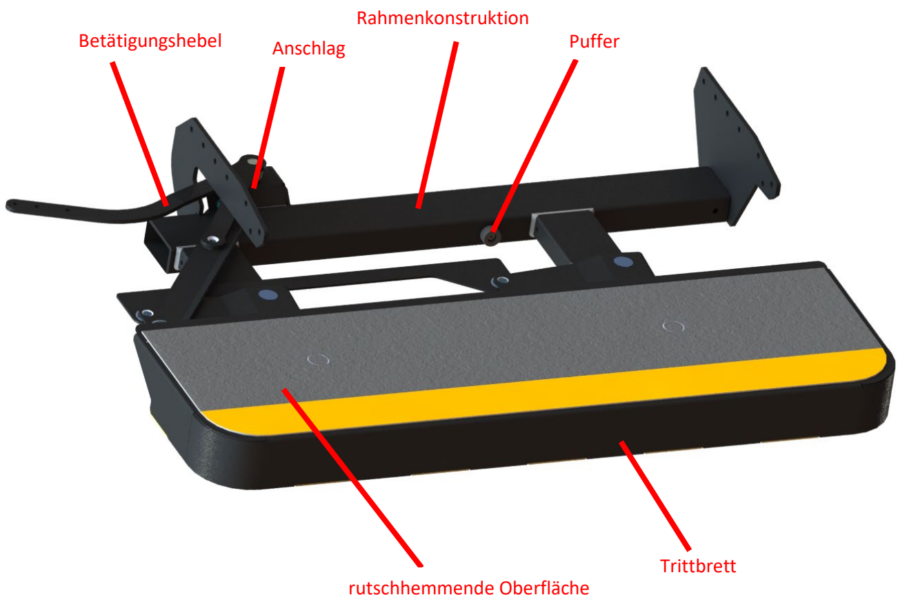
ABBILDUNG 1: AUFBAU TRITTSTUFE
