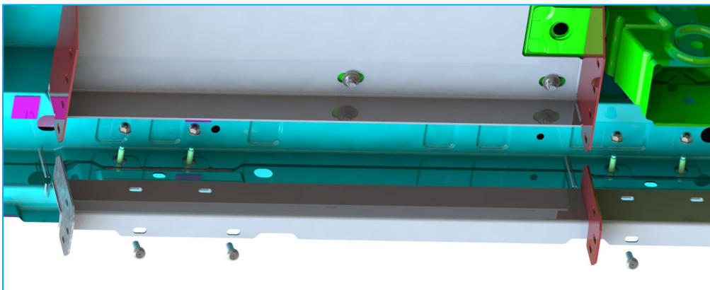
4x Mutter mit Flanschkopf DIN 6926- M8 -N
