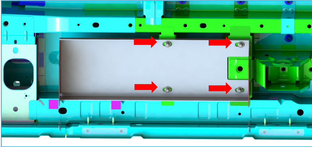
Fertig montierter „Halter hinten“
