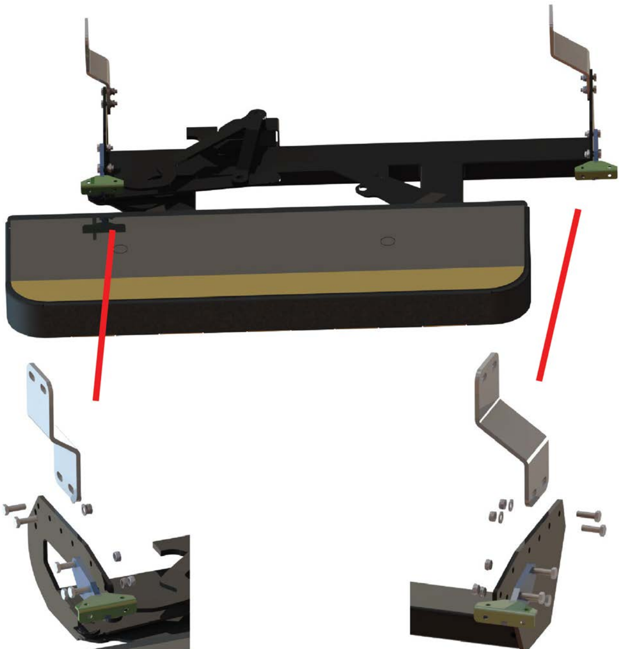
ABBILDUNG 6: VORMONTAGE TRITTSTUFE
