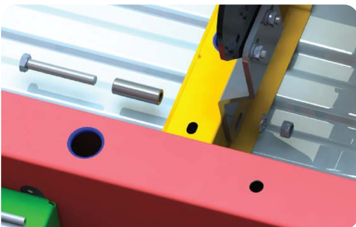
ABBILDUNG 11: VERSCHRAUBUNG TYP 2
