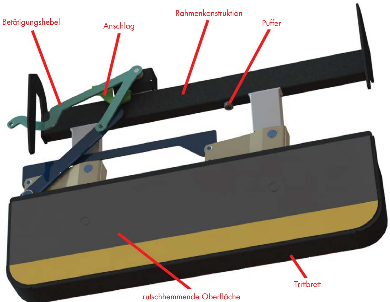
ABBILDUNG 1: AUFBAU TRITTSTUFE
