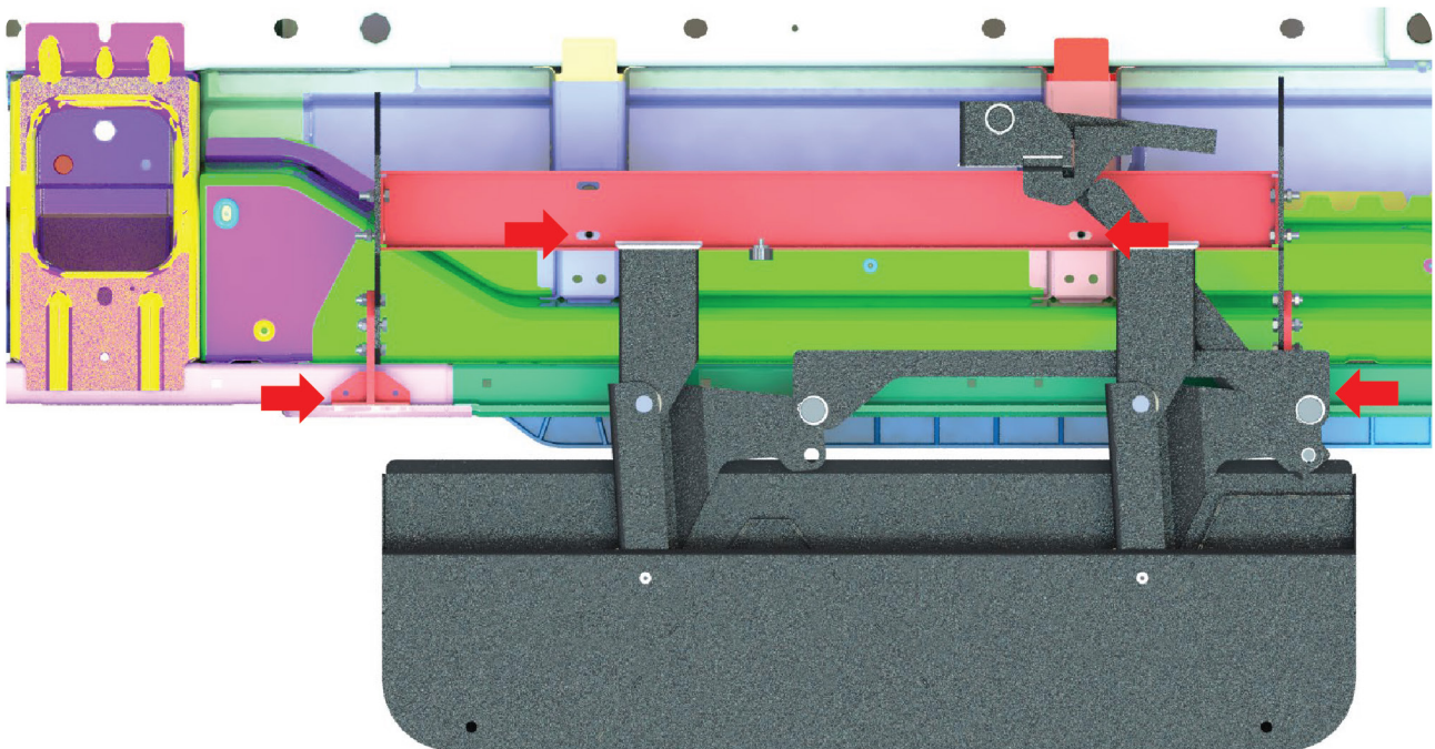
ABBILDUNG 7: X3 STUFE AUSRICHTEN
