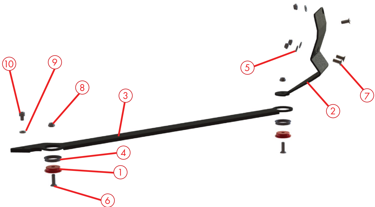
ABBILDUNG 4: TÜRBEFESTIGUNGSSATZ VW CRAFTER /MAN TGE "EXPLOSION"
