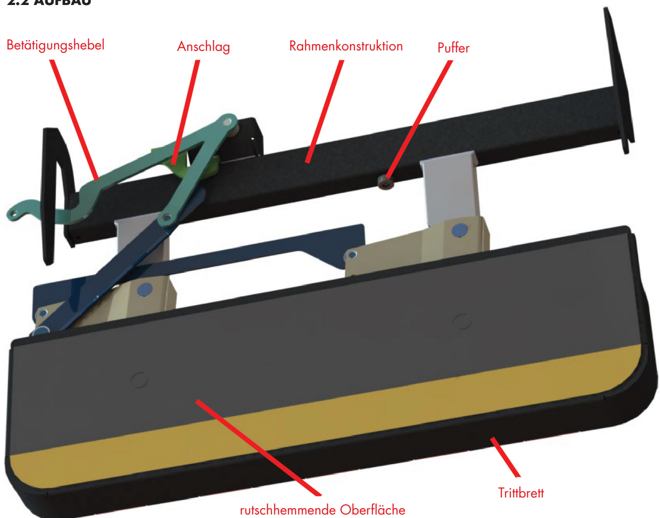
ABBILDUNG 1: AUFBAU TRITTSTUFE
