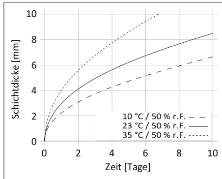
Diagramm 1: Durchhärtegeschwindigkeit Sikaflex®-554
